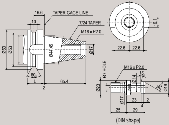
BT40 Unit : mm
