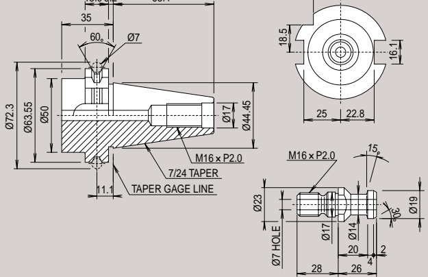
DIN40 Unit : mm
